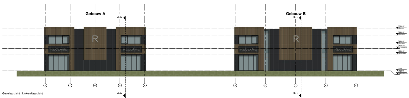
Gevelaanzicht | Linkerzijde
